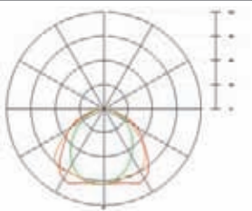
FOTOMETRÍA - PHOTOMETRIC
