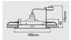
ESQUEMA - SIZES 53
