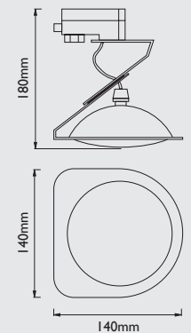
ESQUEMA - SIZES 20202
