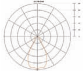
FOTOMETRÍA - PHOTOMETRIC
