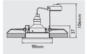
ESQUEMA - SIZES 51
