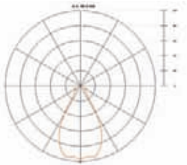
FOTOMETRÍA - PHOTOMETRIC
