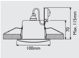
ESQUEMA - SIZES 890
