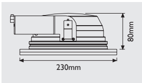
ESQUEMA - SIZES 1930
