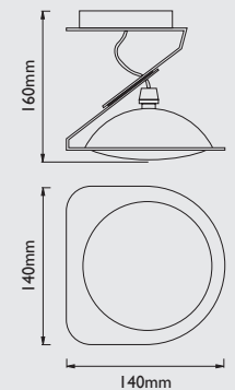
ESQUEMA - SIZES 20200
