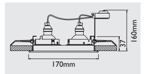
ESQUEMA - SIZES 52
