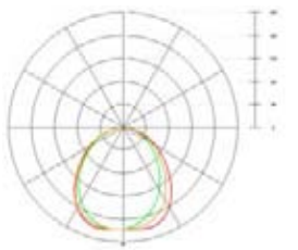
FOTOMETRÍA - PHOTOMETRIC
