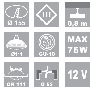
ESQUEMA - SIZES 53
