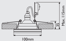
ESQUEMA - SIZES 1922
