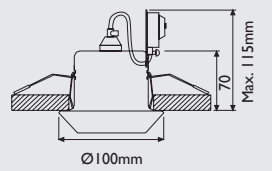
ESQUEMA - SIZES 190
