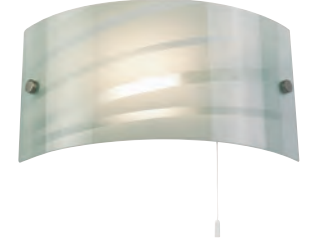
SALSA WALL 96220-WBWH White glass & satin chrome Proj: 105mm H: 165mm W: 310mm 1 x E14
